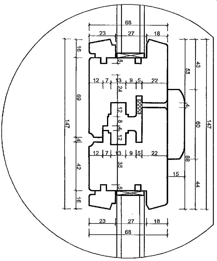
SZCZEGÓL "I" skala 1:2
