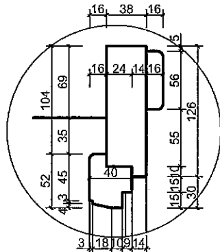
SZCZEGÓŁ "B" skala 1:5
