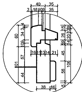
SZCZEGÓŁ "C" skala 1:5
