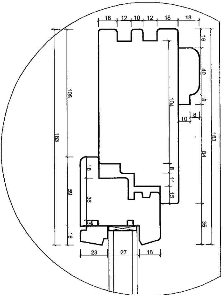
SZCZEGÓŁ "A" skala 1:2
