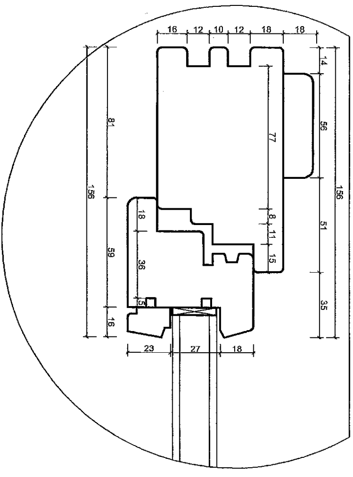
SZCZEGÓL "K" skala 1:2
