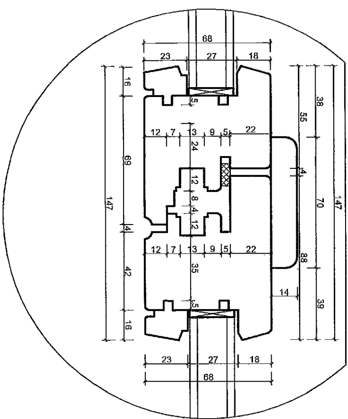
SZCZEGÓŁ "B" skala 1:2
