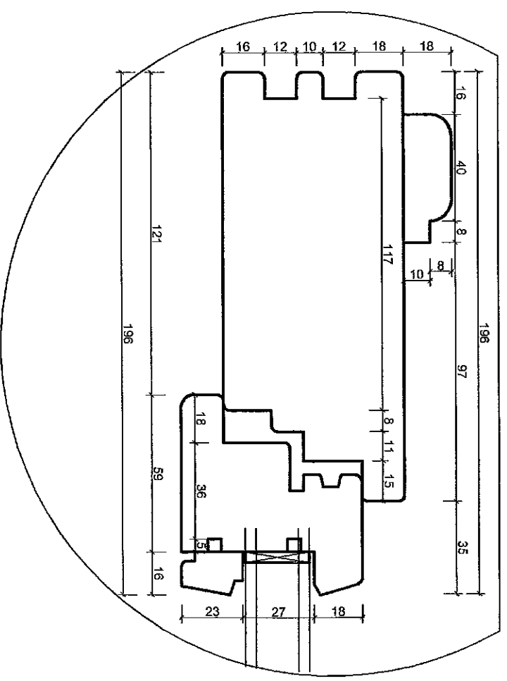
SZCZEGÓŁ "F" skala 1:2
