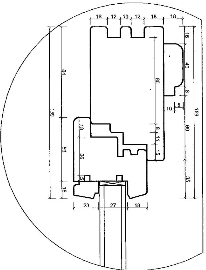
SZCZEGÓŁ "E" skala 1:2
