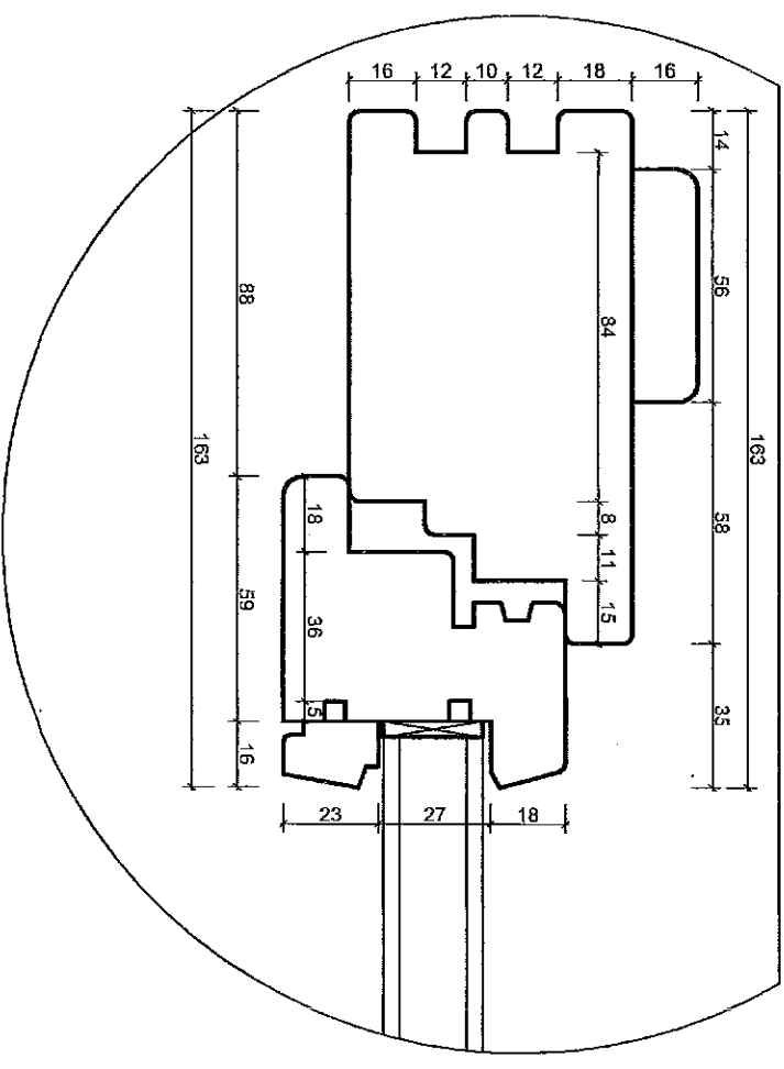
SZCZEGÓL "G" skala 1:2
