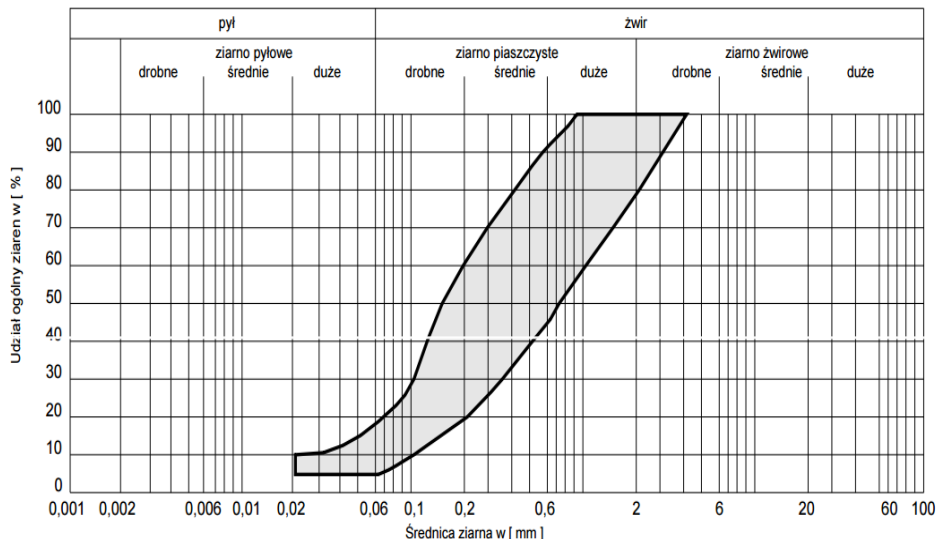
Krzywa uziarnienia gleby darniowej
