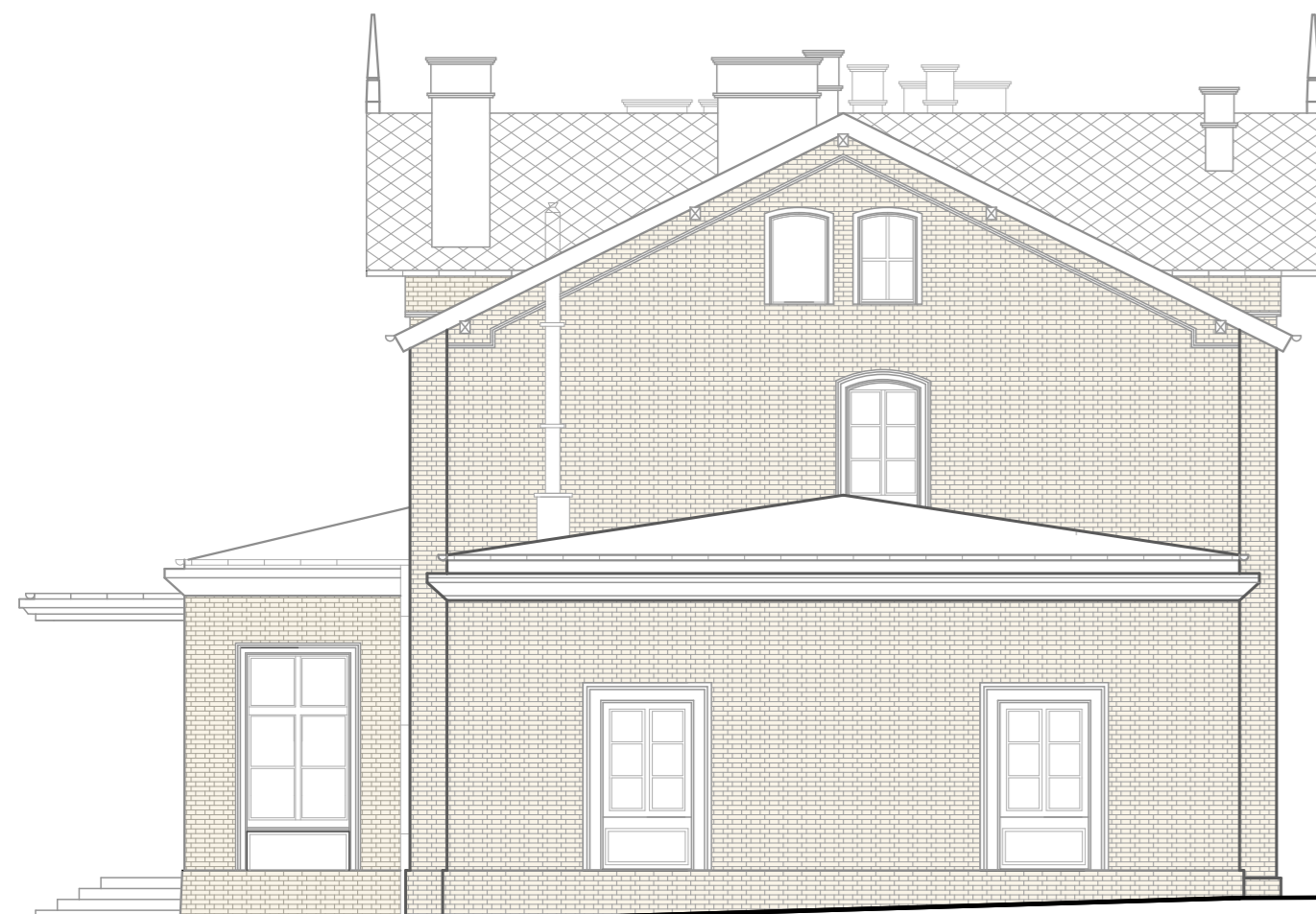
ELEWACJA WSCH - PN 1:100
